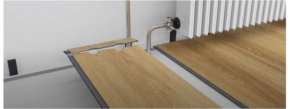
Tuberías: Mida el diámetro y perforo un agujero 12mm. más grande. Corte un trozo, y ponga la pieza recortada en su lugar. / Holes for pipes: Measure the diameter of the pipe and drill a hole that 12mm/1/2" larger. Saw a piece and lay the plank in place on the floor. Then lay the sawed piece in place.
